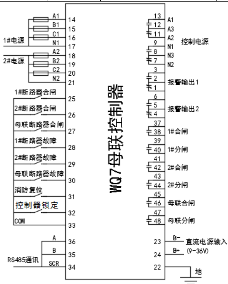
应用原理图
